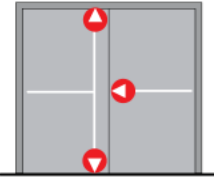
Çift kanat - 3 noktadan kilitleme
